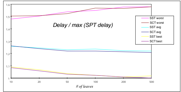
Figure 7 : SST et SCT delays
